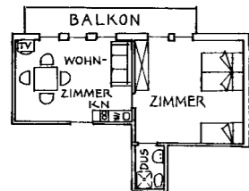
APPARTEMENT Nr. 7 + 19 (41 m 2 ) Wohnraum, Schlafraum, Kochnische, DU/WC und Balkon
