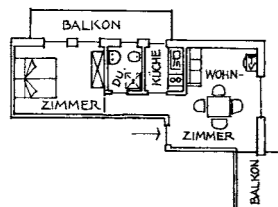
APPARTEMENT Nr. 16 (41 m 2 ) Wohnraum, Schlafraum, Küche, DU/WC und Balkon
