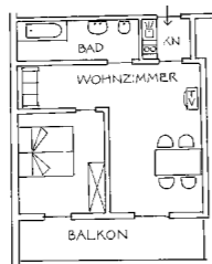
APPARTEMENT Nr. 8 + 9 (39 m 2 ) Wohnraum, Schlafraum, Kochnische, Bad/WC und Balkon
